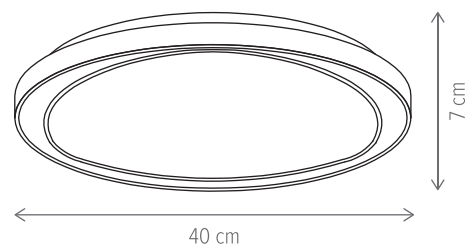
Saturnus Uranus
