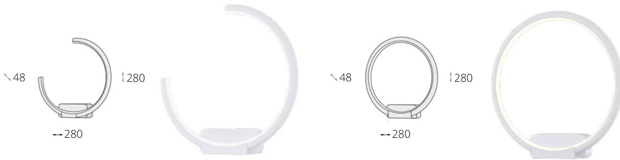
▲ MOD877WL-L13W ☞ LED 13W H: 280, W: 280, L: 48 mm, 800 Lumen, 3000 K, 80 RA, 120 °, 220-240 V, IP20
