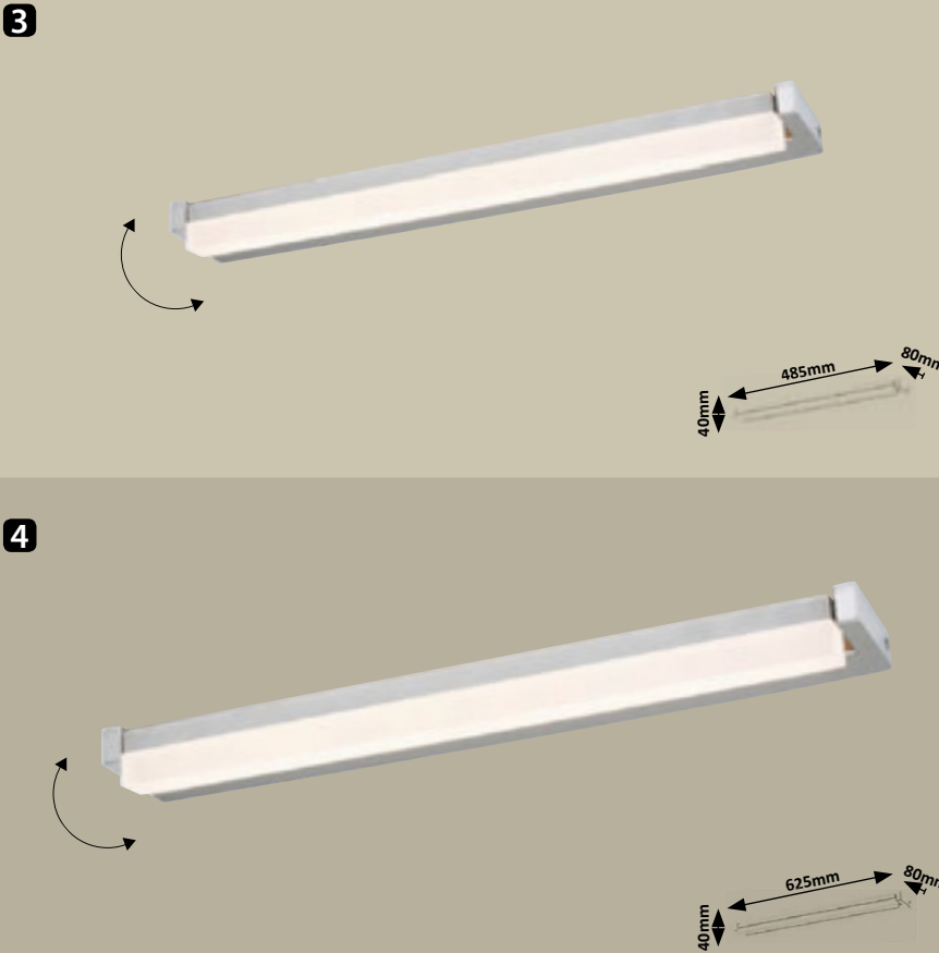
3 I446 M P • LED / 8W (705lm, 3000K) incl. IP20 chrome
