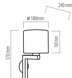
3096 TROY 1 x E27 max 60W AB 8838
