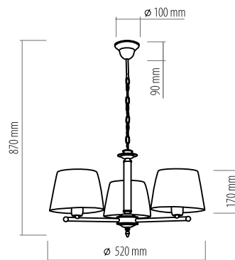
1105 QUEEN 5 x E27, max 60W AB 8263
