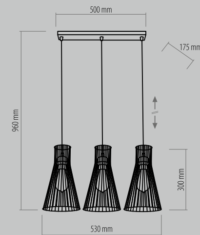
1501 VITO WHITE 3 x E27, max 60W DM 19
